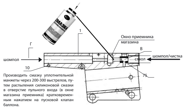
Рисунок А6 – Схема обслуживания уплотнительной манжеты
