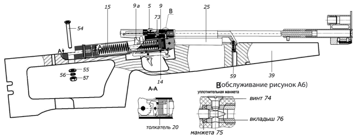
Рисунок А3 – Схема механизмов винтовки
