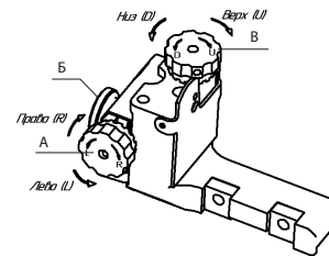
Рисунок А7 – Схема регулировки диоптрического прицела
